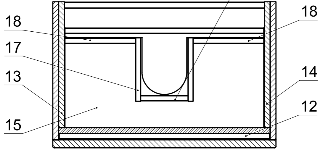
C-C (1 : 7)
