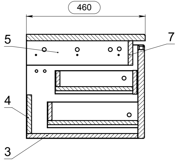
B-B (1 : 7)
