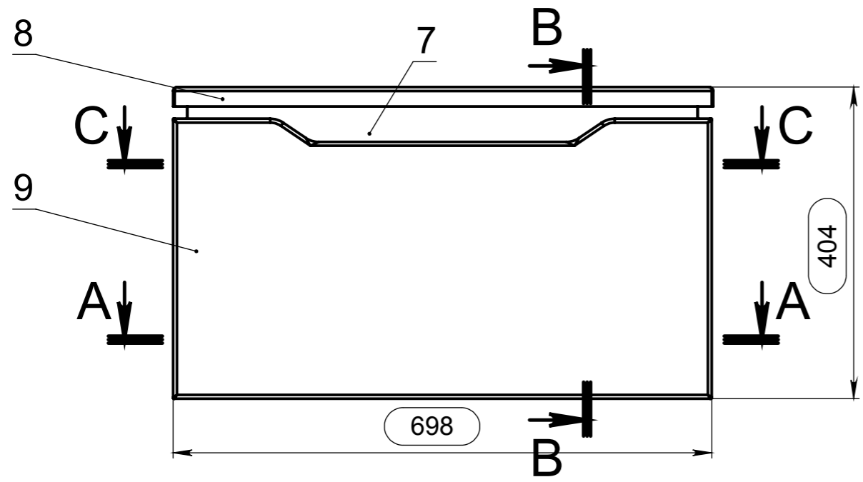
A-A (1 : 7)
