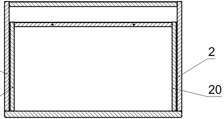
C-C (1 : 7)
